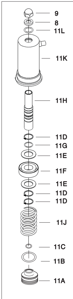
Type 10 Actuator
