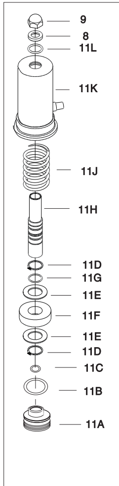
Type 20 Actuator
