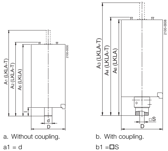
Fig. 2. Dimensions - actuator.
